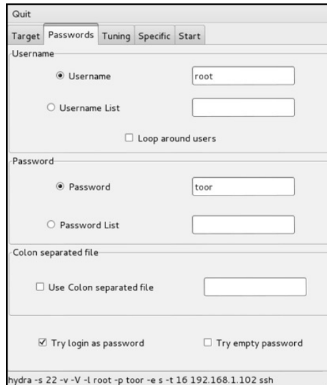
Figura 11.3 – Tela de seleção password.
